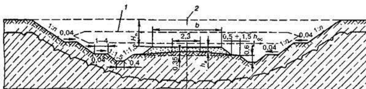
Рисунок 20.6 - Схема устройства насыпи над подземным льдом, залегающим на глубине, равной мощности деятельного слоя
