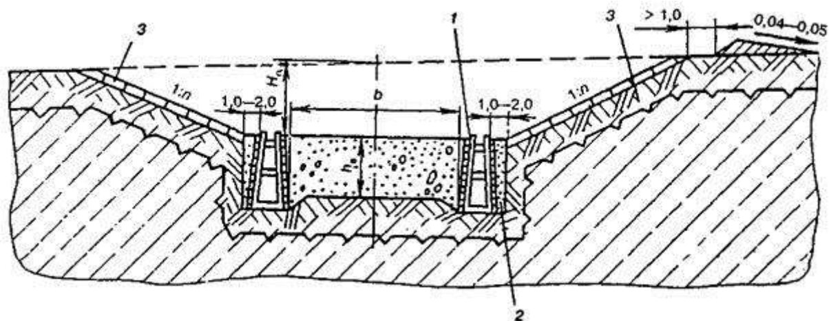
Рисунок 20.4 - Поперечный профиль выемки в глинистых грунтах, переходящих при оттаивании в текучепластичное и текучее состояние
