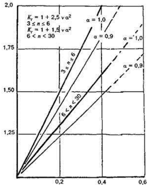
Рисунок Р.4 - График для определения коэффициента безопасности по грунту K_r в зависимости от коэффициента вариации v ряда измерений и заданной надежности \alpha .
