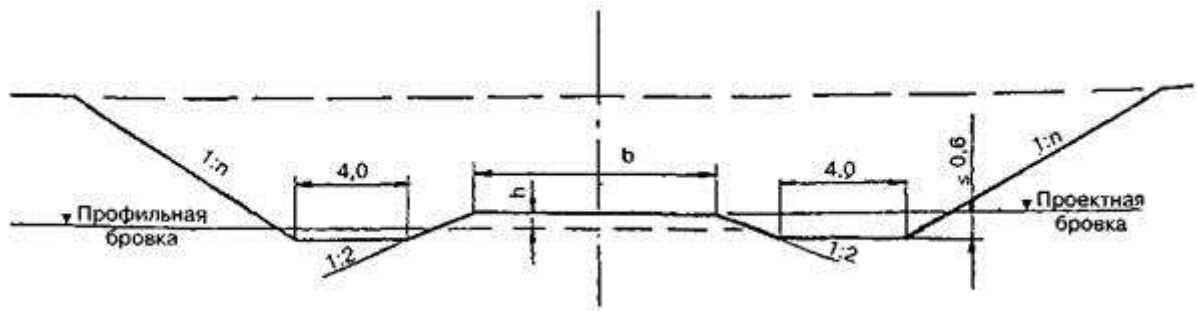
Рисунок 10.4 - Поперечный профиль выемки в песках на сильноэрозийных участках с кювет-траншеями
