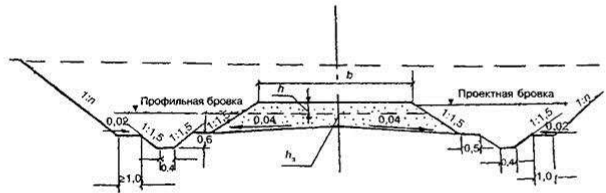
Рисунок 10.6 - Поперечный профиль выемки глубиной (высотой верхнего откоса) до 12 м в глинистых тугопластичных грунтах ( 0,25 < I_L < 0,50 )
