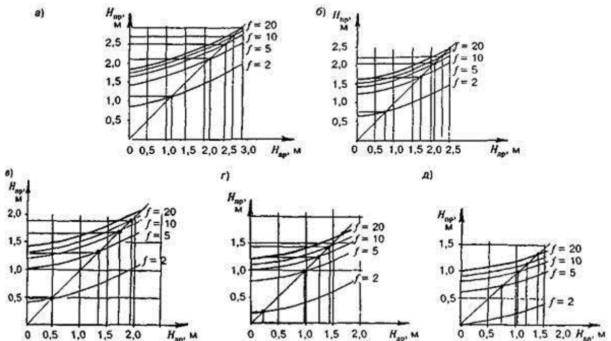
a - при многолетней средней сумме градусо-суток отрицательных температур наружного воздуха \Omega , °C·сут - 2600; б - то же \Omega - 2200; в - то же \Omega - 1800; г - то же \Omega - 1400; д - то же \Omega - 1000
