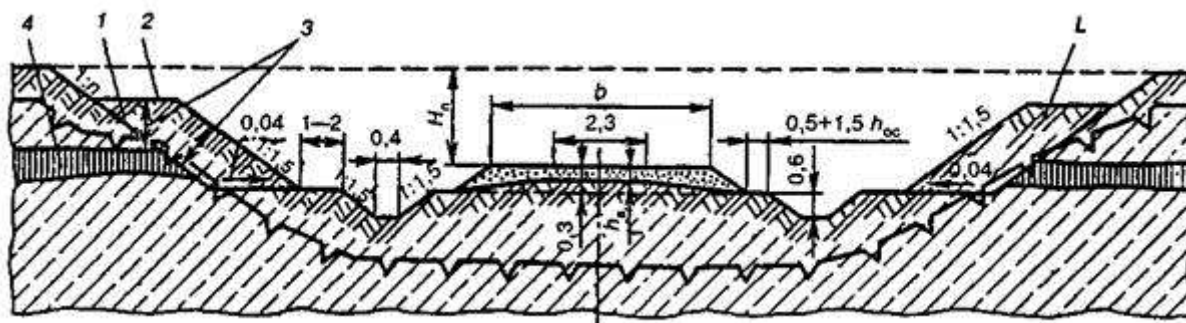
Рисунок 20.7 - Поперечный профиль выемки, прорезающей линзу льда
