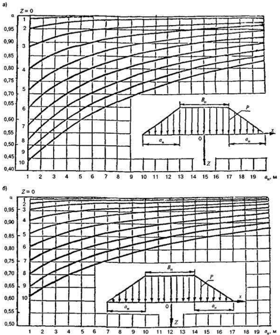
Рисунок Е.1 - Значения коэффициента \alpha в основании насыпи в зависимости от Z и a_n
