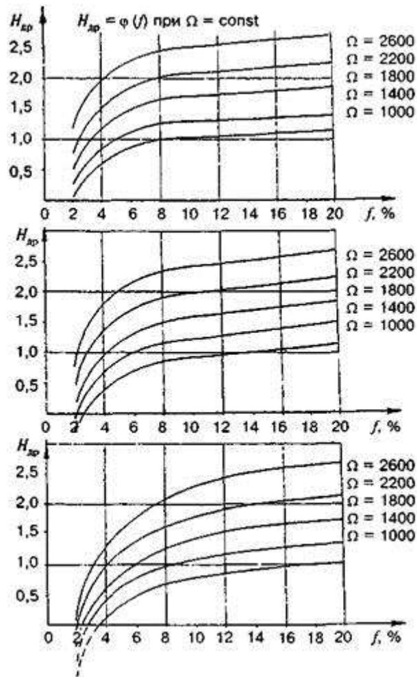
Рисунок В.1 - Графики для определения толщины слоя дренирующего грунта, обеспечивающего не превышение допустимой величины пучения 20 мм, при различной интенсивности пучения f , %, для различных климатических условий
