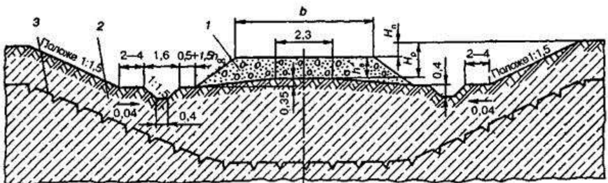
Рисунок 20.2 - Схема устройства искусственного основания насыпей высотой менее 1 м на участках с вечномерзлыми грунтами II и III категорий (а) и IV категории просадочности (б)
