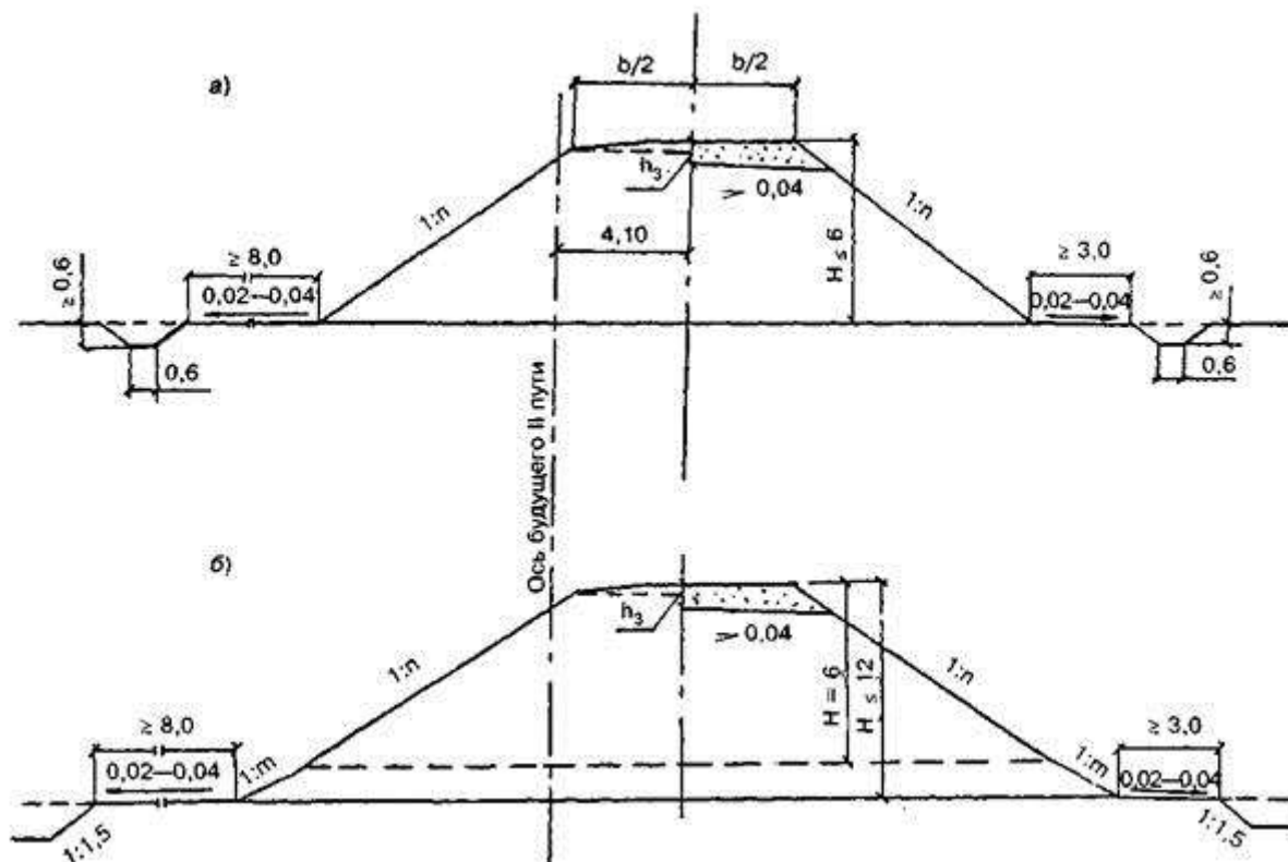
a - насыпь без защитного слоя H \leq 6 м; б - то же, высотой от 6 до 12 м; в - насыпь с защитным слоем H \leq 6 м; г - то же, высотой от 6 до 12 м
