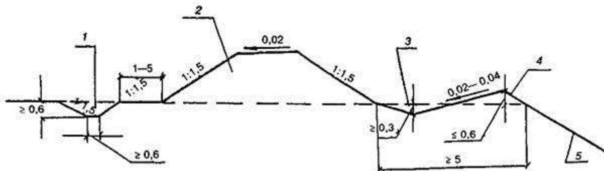
Рисунок 16.1 - Схема размещения банкетов, кавальеров, забанкетных и нагорных канав
