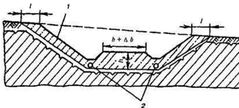
Рисунок 20.3 - Поперечный профиль выемки в тугопластичных и мягкопластичных глинистых грунтах
