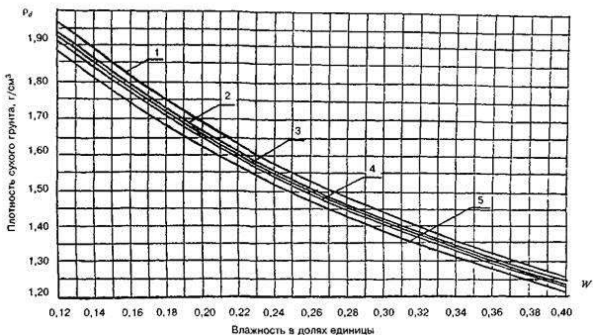
Рисунок 4.1 Зависимость возможного уплотнения грунта от его естественной влажности
