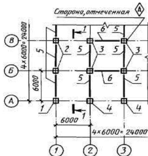
Схема расположения колонн, ригелей и балок перекрытия на отм...
