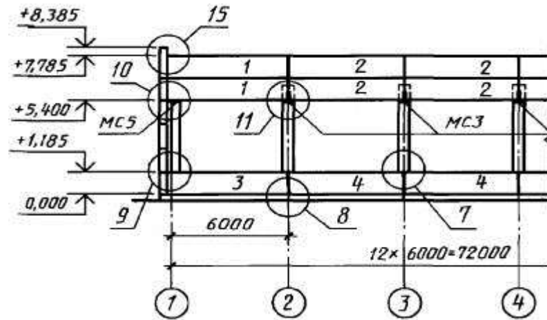
Схема расположения панелей стен, перегородок и других элементов жилого дома
