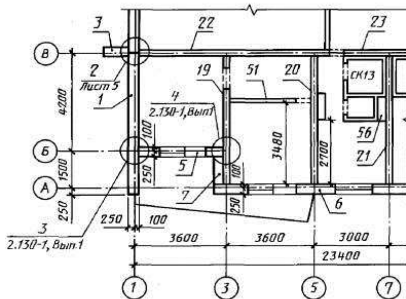
Схема расположения колонн, ригелей и балок перекрытия на отм...
