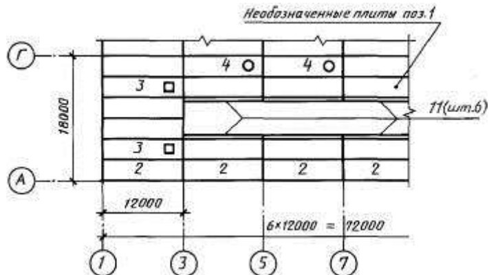
Схема расположения плит покрытия
