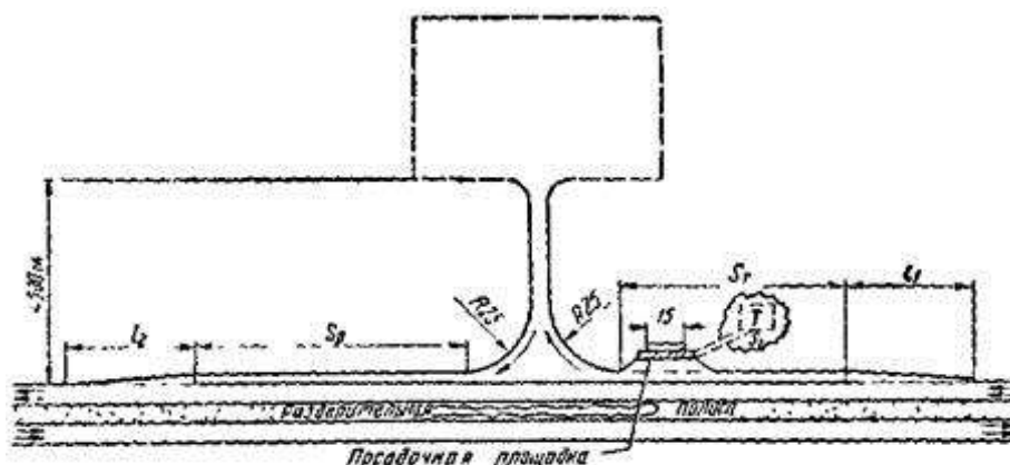
Рис. 9. Пример (схема) размещения площадок различных сооружений на общих с автобусной остановкой полосах торможения и разгона.
