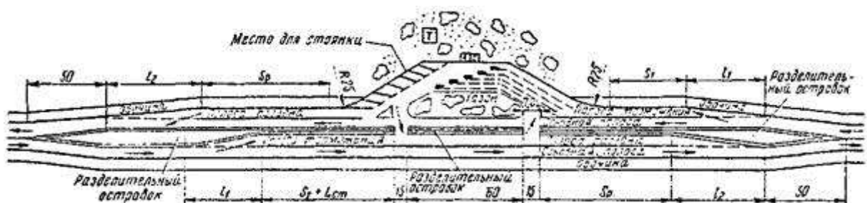
Рис. 7. Пример (схема) размещения автозаправочной станции на дороге II категории при интенсивности до 4000 автомобилей в сутки и на дороге III категории.
