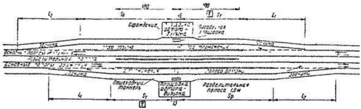
Рис. 4. Пример (схема) размещения автобусных остановок на дороге I категории (то же, II категории)
