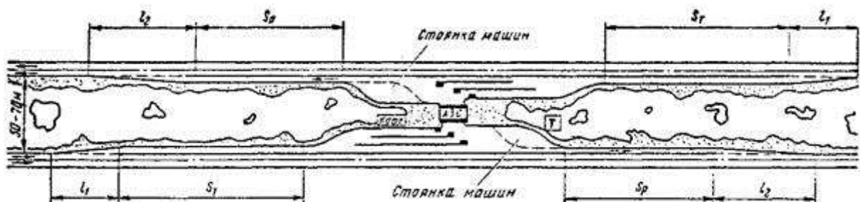
Рис. 6. Пример (схема) основного размещения автозаправочной станции на дороге I категории.
