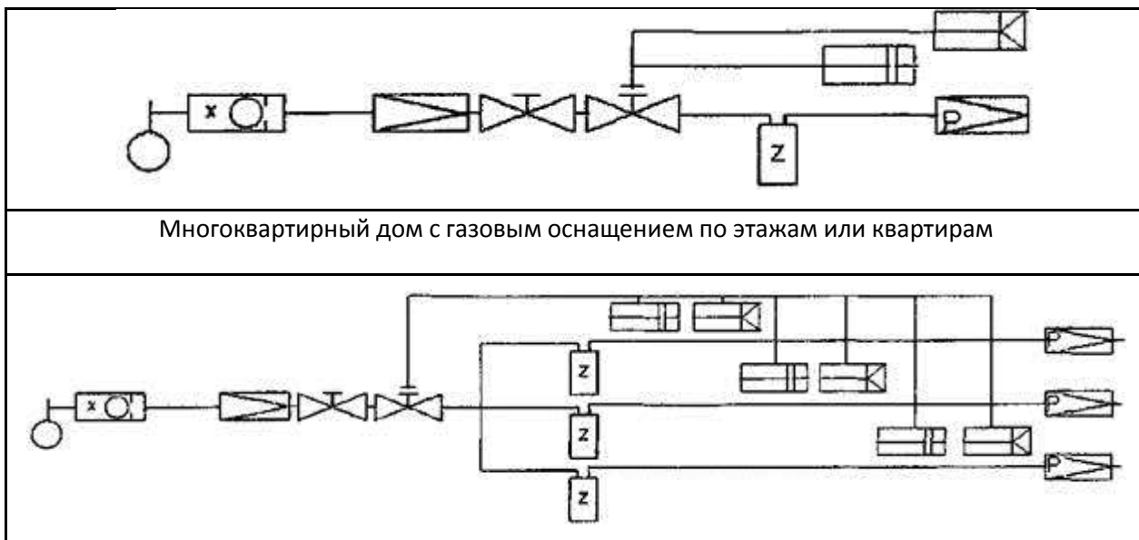
Рисунок Д.2 - Активные меры безопасности при давлении в наружном газопроводе выше 0,005 МПа до 0,6 МПа включительно и приборы, регулирующие давление газа
