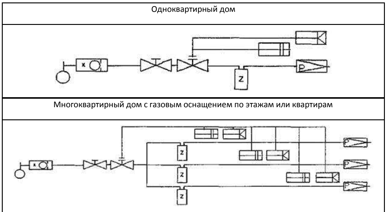
Рисунок Д.1 - Активные меры безопасности при давлении в наружном газопроводе выше 0,0025 МПа до 0,005 МПа включительно и приборы, регулирующие давление газа
