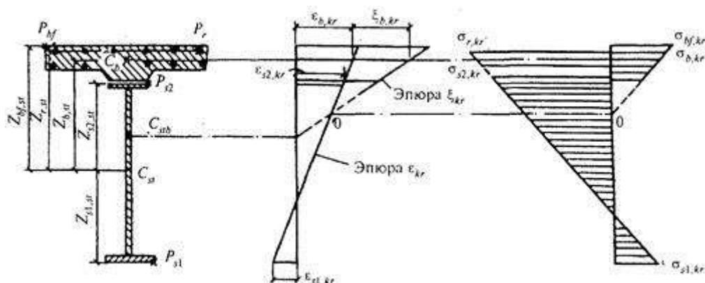
Рисунок Ш.1 - Эпюры относительных деформаций и внутренних напряжений от ползучести бетона
