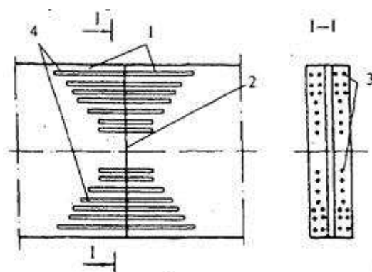
Рисунок 10.1 - Клеештыревой стык
