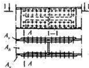
Рисунок Ц.4 - Расположение проверяемого на выносливость расчетного сечения А-А по основному металлу в сечении брутто по первому ряду высокопрочных болтов в прикреплении к узлу или в стыке двухстенчатых элементов
