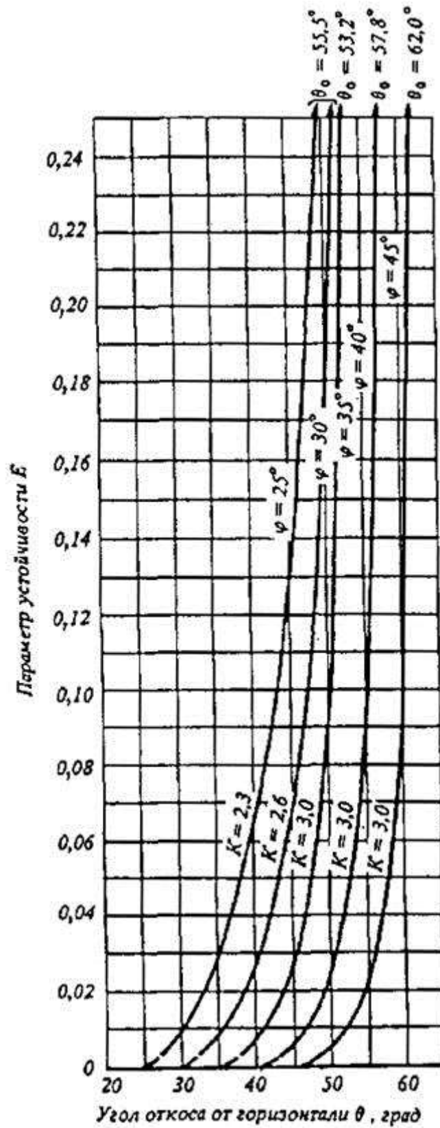
Черт. 4. Графики для определения крутизны откоса при 2 < K < 3
