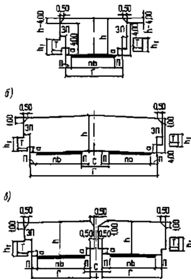
Черт. 1. Схемы габаритов приближения конструкций на автодорожных и городских мостах
