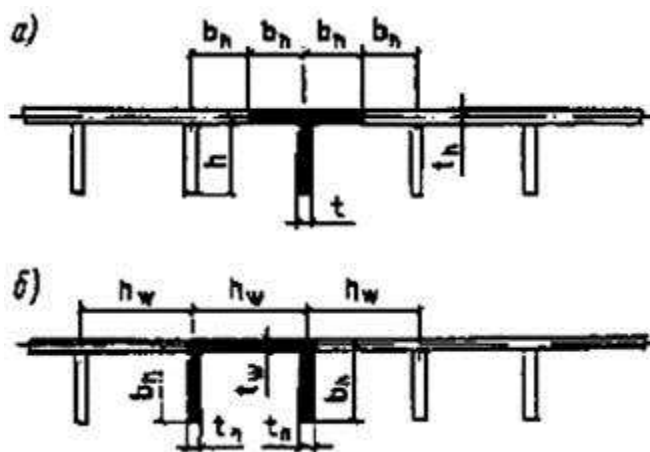
Черт. 12. Схемы расчетных сечений пластинок ортотропных плит
