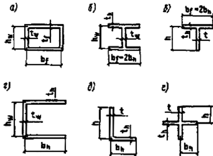
Черт. 11. Схемы расчетных сечений элементов, не подкреплённых ребрами жесткости
