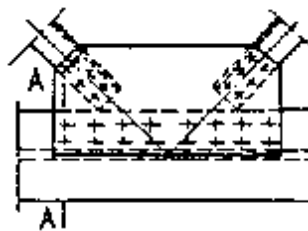
Черт. 3. Расположение проверяемого на выносливость расчетного сечения А-А по основному металлу в сечении брутто по первому ряду высокопрочных болтов в прикреплении фасонки к нестыкуемым в данном узле поясам сплошных балок и элементам решетчатых форм
