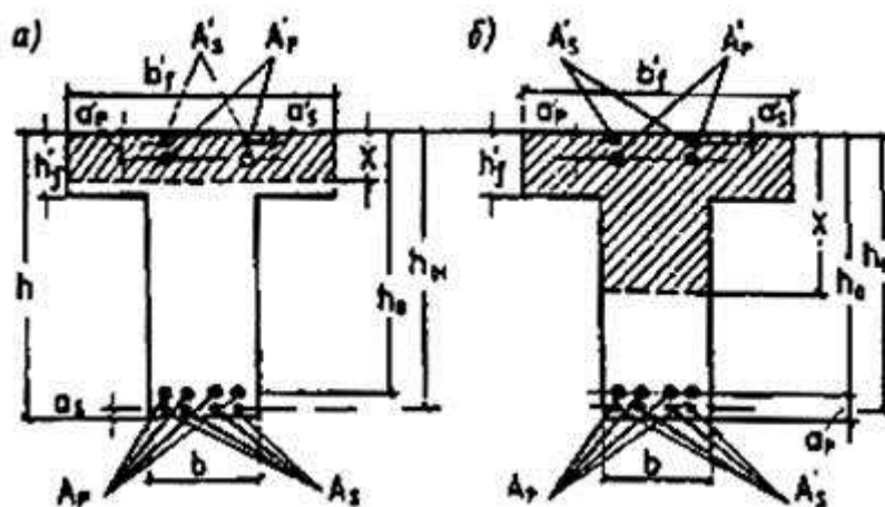
Черт. 3. Форма сжатой зоны в сечениях железобетонных элементов с плитой в сжатой зоне
