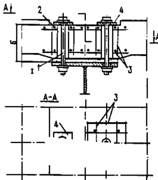
Конструкция болтового объединения
