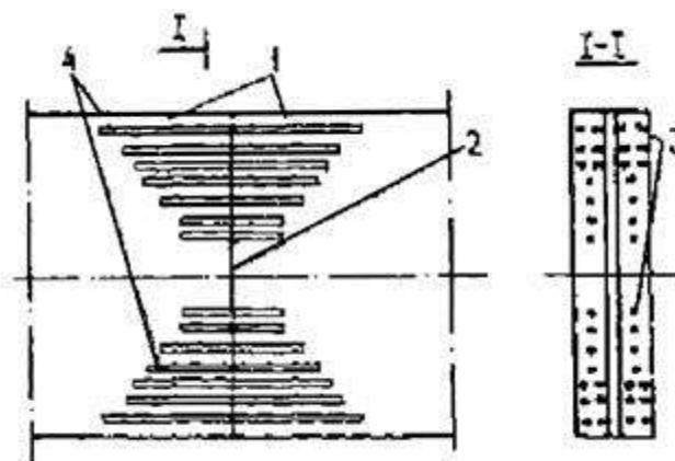
Черт. 18. Клеештыревой стык
