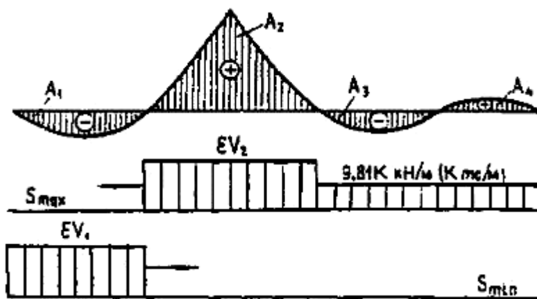
Черт. 5. Схема загрузения участков линии влияния для определения максимальных и минимальных усилий (напряжений) при расчете на выносливость
