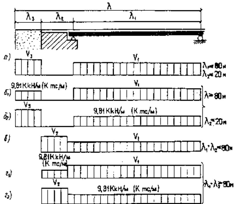
Черт. 3. Схема загрузки участков линии влияния при \lambda > 80 м
