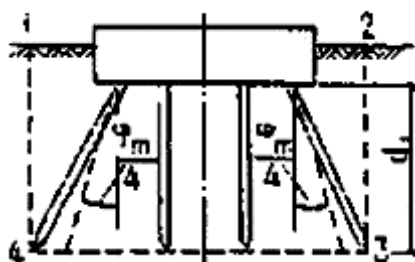
Черт. 2. Условный свайный фундамент с ростверком, заглубленным в грунт при угле наклона свай более \varphi_m/4
