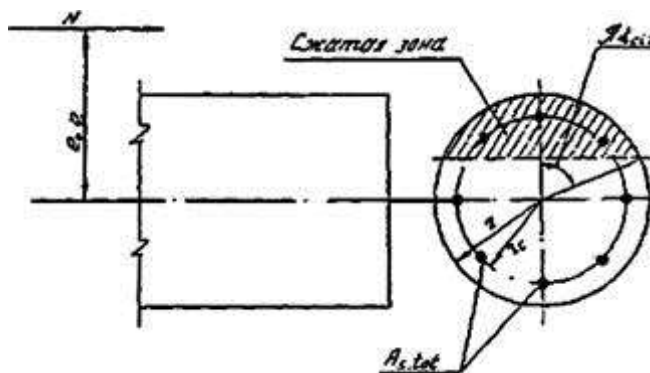
Чертеж. Схема, принимаемая при расчете круглого сечения внецентренно сжатого элемента
