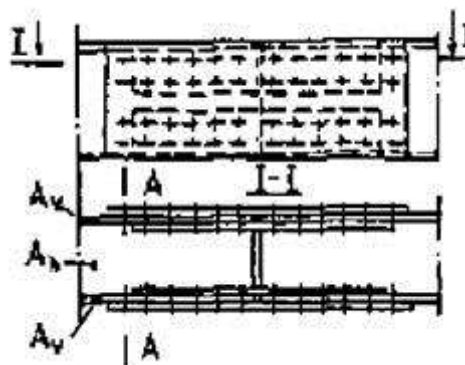
Черт. 3. Расположение проверяемого на выносливость расчетного сечения А-А по основному металлу в сечении брутто по первому ряду высокопрочных болтов в прикреплении фасонки к нестыкуемым в данном узле поясам сплошных балок и элементам решетчатых форм
