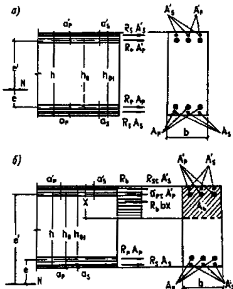
Черт. 6. Схема усилий и эпюра напряжений в сечении, нормальном к продольной оси внецентренно растянутого железобетонного элемента, при расчете его по прочности
