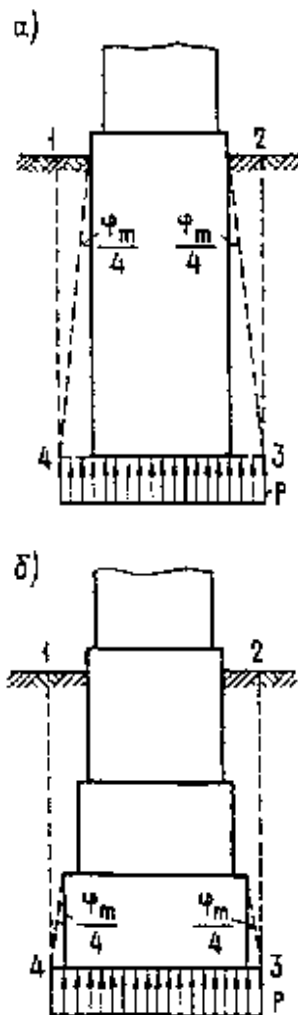
Черт. 5. Условный фундамент из опускного колодца
