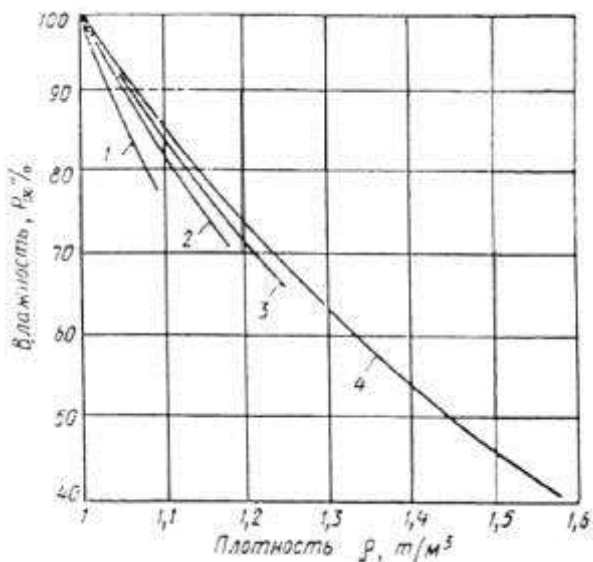
Рис. 5. Значения плотности в зависимости от влажности осадка станции осветления и обезцвечивания воды
