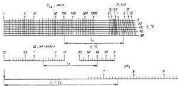
Рис. 1. Номограмма для определения pH насыщения воды карбонатом кальция (pH с )
