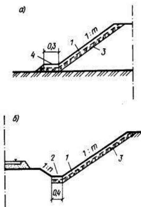
Рис. 63. Схема укрепления неподтопляемых откосов механизированным гидропосевом трав
