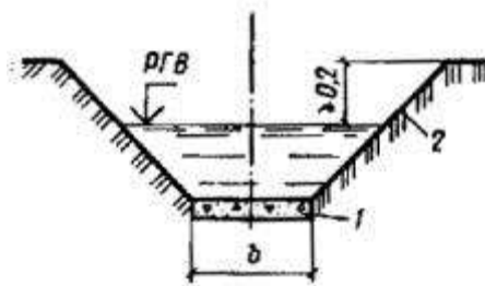
Рис. 60. Укрепление дна канав щебнем и обсевом откосов семенами дикорастущих трав 1 - щебень с песком слоем толщиной 0,08 - 0,1 м; 2 - откос, засеянный семенами дикорастущих трав; РГВ - расчетный горизонт воды
