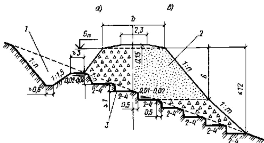
Рис. 5. Конструкции насыпей
