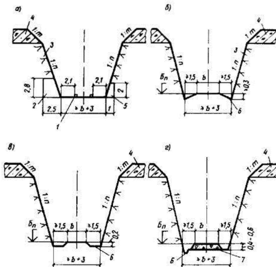
Рис. 25. Конструкция выемки в слабовыветривающихся скальных грунтах
