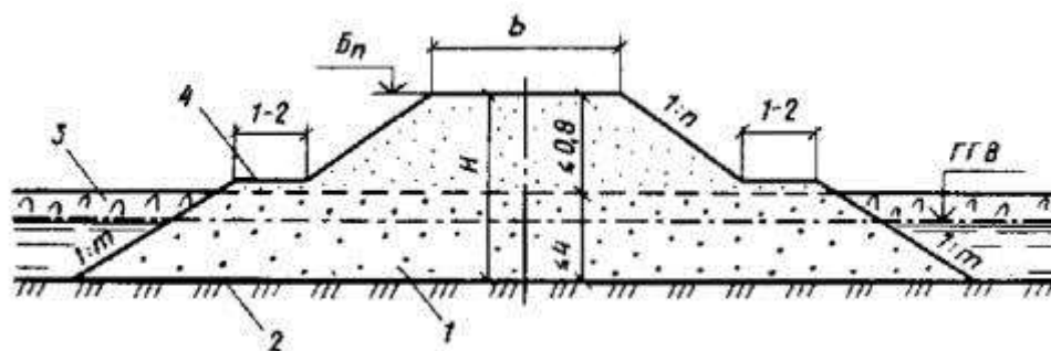
Рис. 11. Конструкция насыпи на болоте III типа со славвиной, глубиной более 4 м, из дренирующих грунтов высотой более 0,8 м
