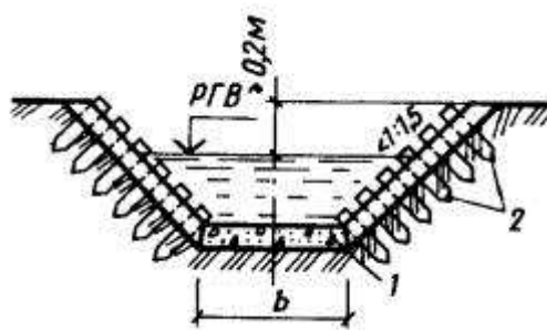
Рис. 59. Укрепление дна канав щебнем и одерновкой откосов
