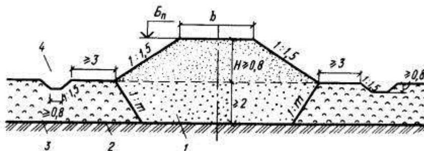
Рис. 9. Конструкция насыпи высотой до 3 м на болоте I типа, глубиной до 2 м, из дренирующих грунтов
