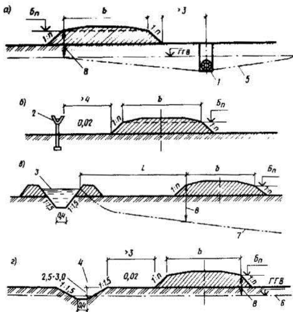
Рис. 27. Конструкция насыпи вблизи ирригационных сооружений
