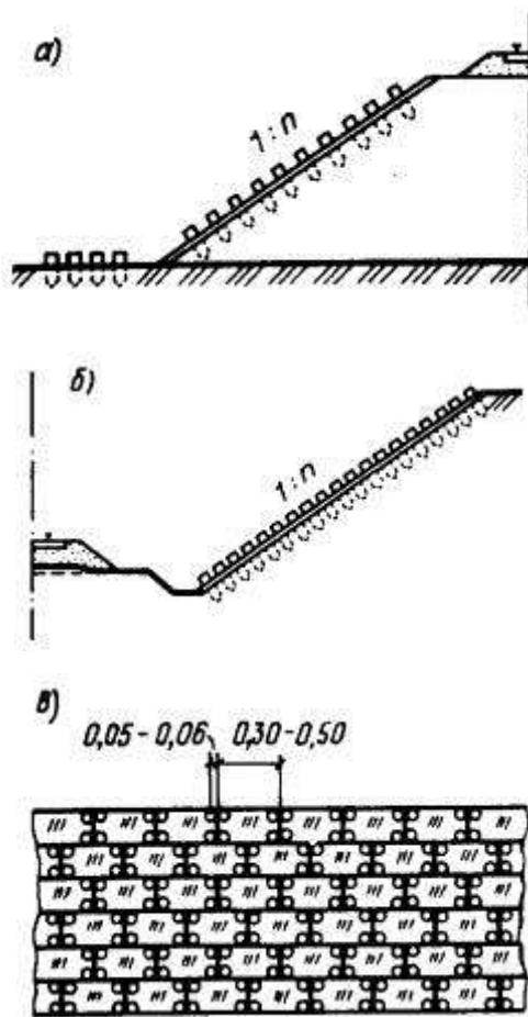
Рис. 61. Укрепление откосов одерновкой плашмя а - неподтопляемой насыпи; б, в - схемы крепления дернин деревянными кольями
