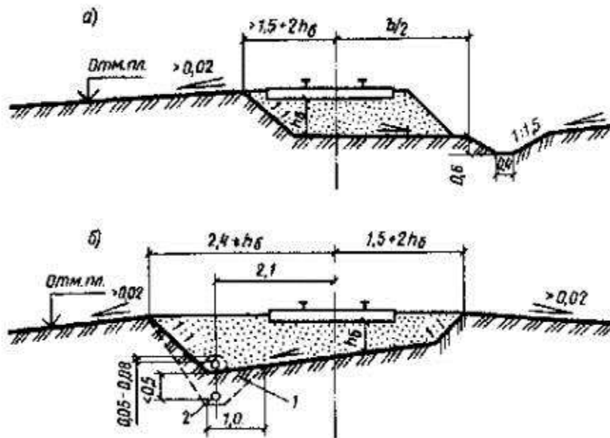
Рис. 2. Конструкции земляного полотна
