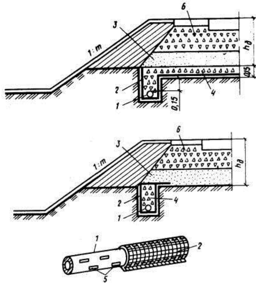
Рис. 101. Конструкции дренажей мелкого заложения с использованием геотекстиля 1 - асбоцементная труба; 2 - геотекстиль; 3 - песок мелкий с коэффициентом фильтрации не менее 2 м/сут; 4 - щебень; 5 - щели в трубе; 6 - щебень подстилающего слоя; h_d - мощность слоя дорожной одежды
