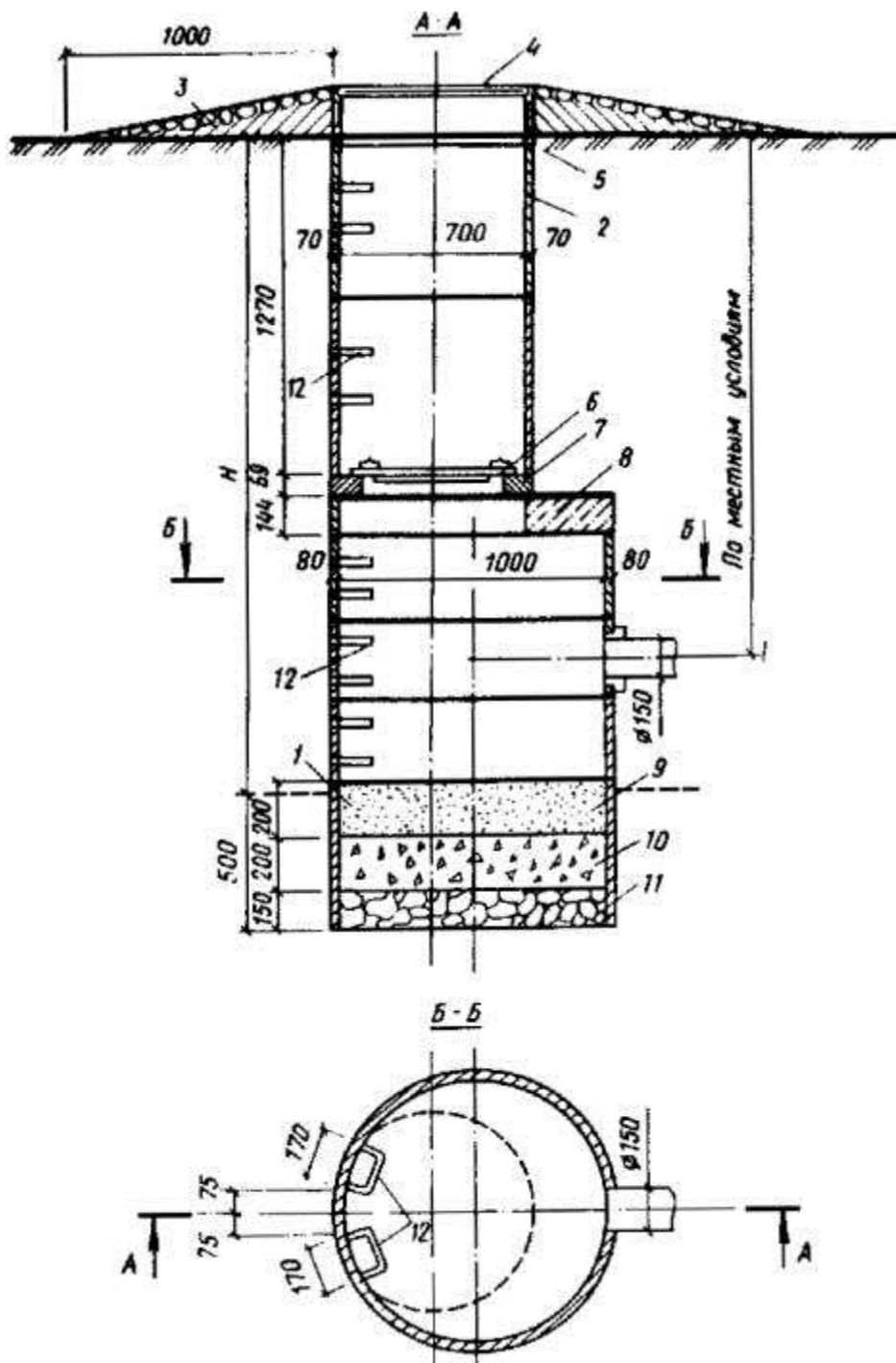
Рис. 56. Конструкция поглощающего колодца из железобетонных колец диаметром 0,7 и 1
