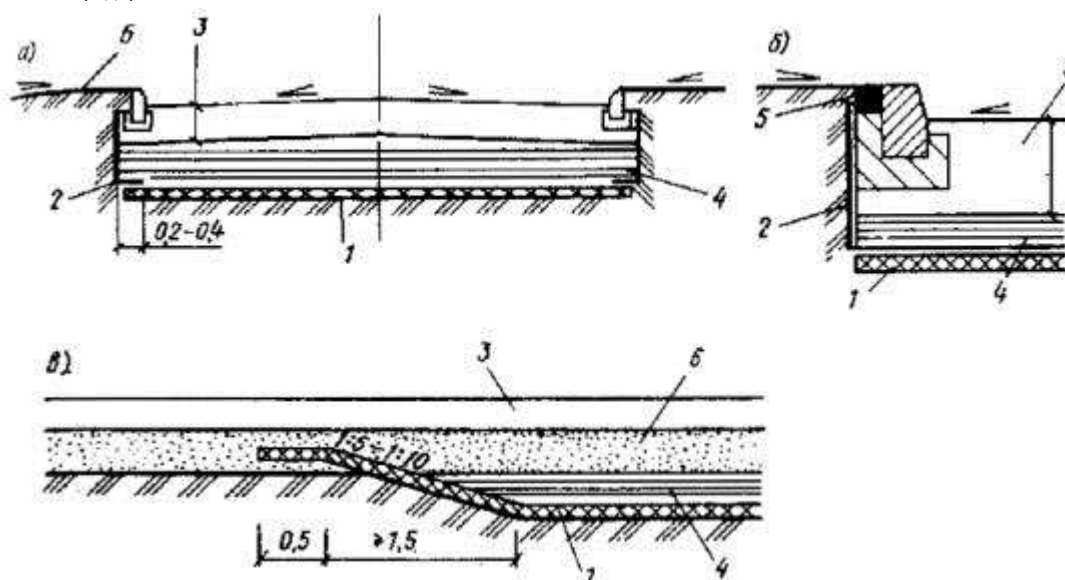
Рис. 103. Устройство гидроизоляции
