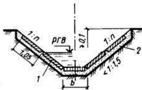
Рис. 62. Конструкция крепления канавы железобетонными плитами
