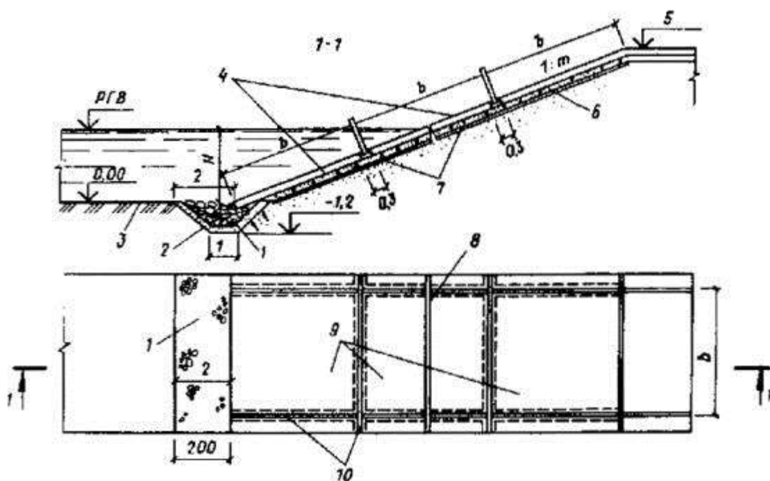
Рис. 67. Укрепление подтопляемых откосов монолитными железобетонными плитами 1 - упорная призма из камня; 2 - песок крупнозернистый; 3 - поверхность дна водоема; 4 - плиты железобетонные; 5 - отметка верха крепления откоса; 6 - подстилающий слой из щебня и гравия; 7 - плиты сборные железобетонные; 8 - температурно-усадочный шов; 9 - плиты железобетонные монолитные; 10 - конструктивные швы; PГВ - расчетный горизонт воды; b - ширина плиты
