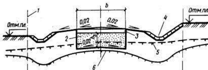
Рис. 94. Конструкция земляного полотна дорог на застраиваемой территории, на грунтах III и IV категории термпросадочности с заменой на дренирующий грунт
