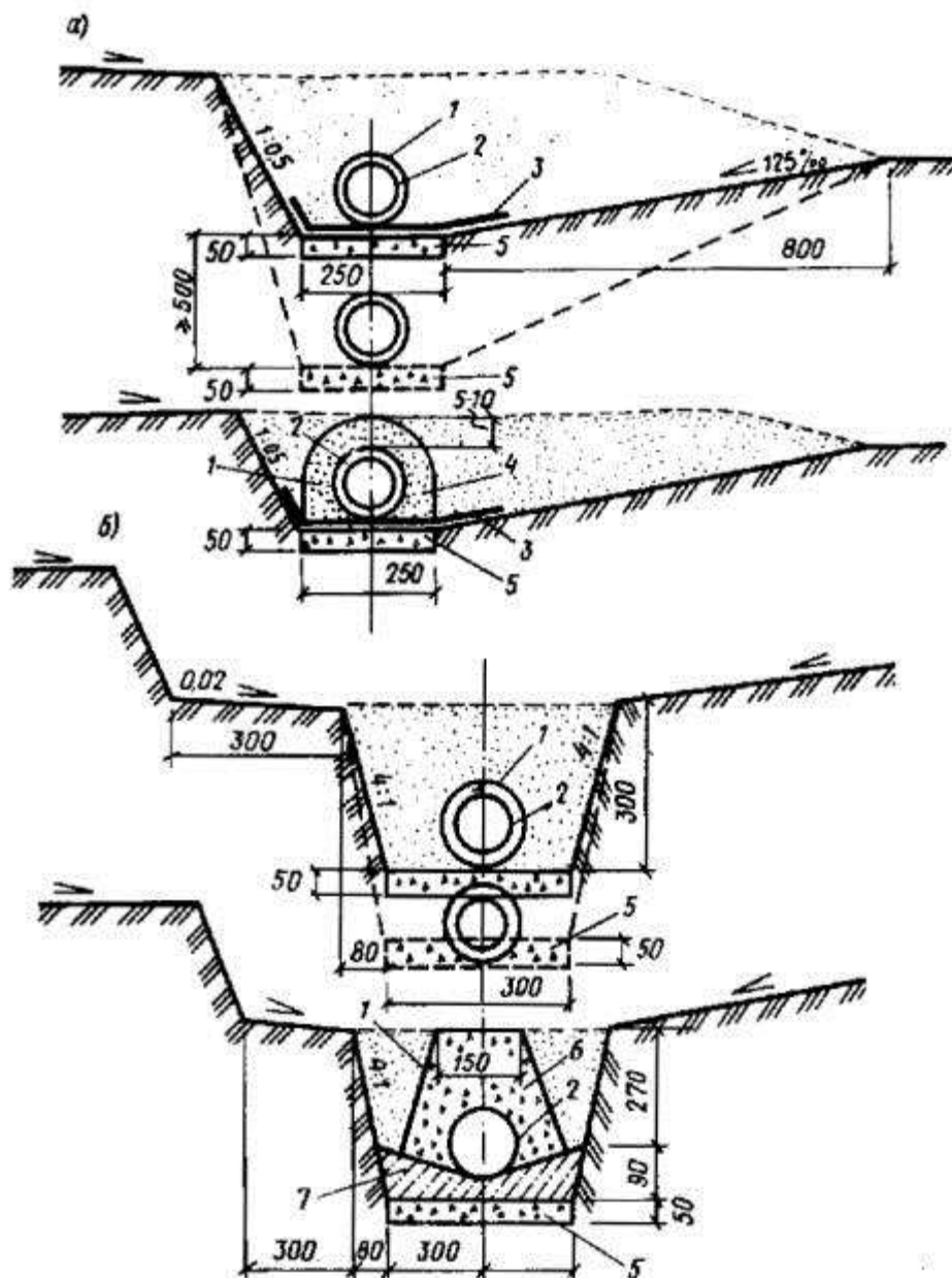
Рис. 75. Конструкции железнодорожных путевых дренажей
