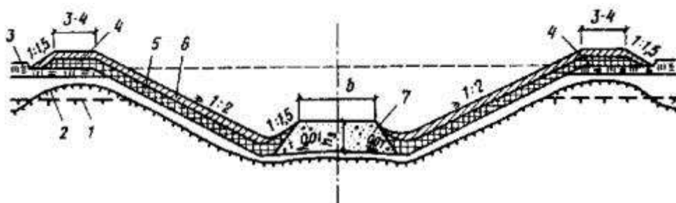
Рис. 37. Конструкция выемки глубиной до 6 м на вечномерзлых грунтах III категории термпросадочности с заменой на дренирующий грунт и термоизоляцией откосов пенопластом или торфом
