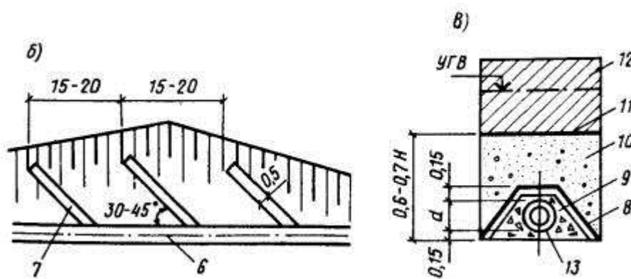
Рис. 102. Конструкция откосного дренажа с применением геотекстиля
