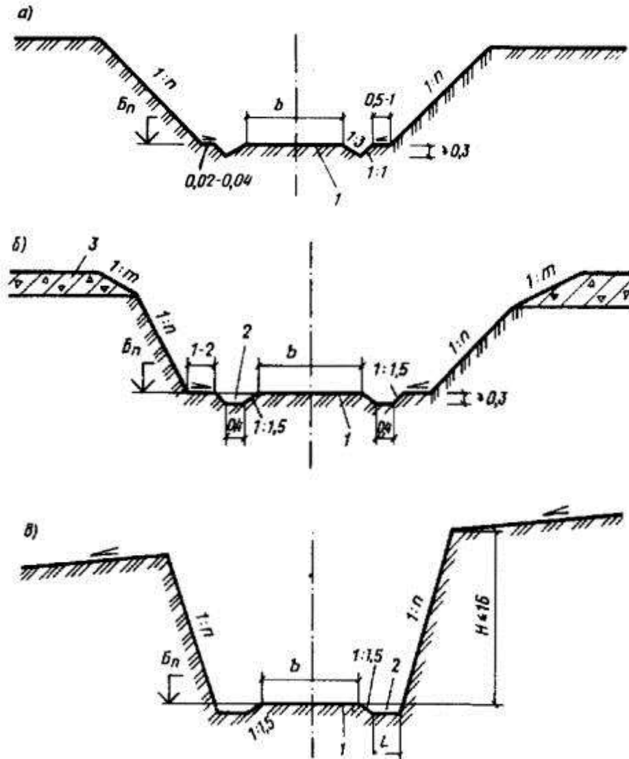
Рис. 20. Конструкции выемок в скальных грунтах
