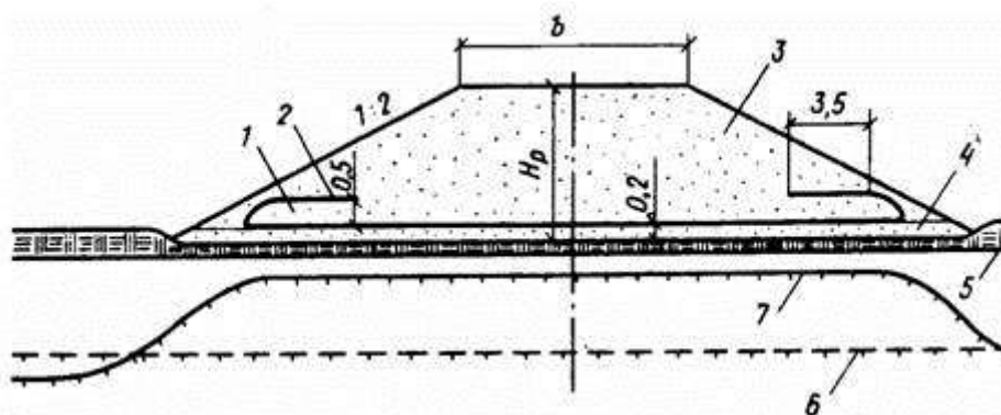
Рис. 91. Конструкция насыпи высотой более 1,5 м на грунтах III категории термопросадочности, из сухих талых сыпуче- или сухомерзлых песчаных грунтов; нижняя часть насыпи заключается в полуобойму из геотекстиля
